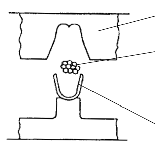
Obermatritze (Crimpstempel) Crimp indenter Abisolierter Leiter, in oder über der Leitercrimphülse positioniert Stripped wire in or above the conductor crimp barrel Offene Crimphülse mit geschragten Außenflanken Open crimp barrel with chambered outer flanks
