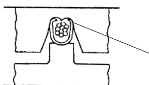
Untermatritze (Amboss) Crimp anvil Obermatritze und die sich einrollenden Crimphülsenflanken zwingen das abisolierte Leiterende in den Crimphülsenboden The indenter and the rolling up crimp flanks force the stripped conductor end into the base of the crimp barrel
