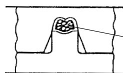
Die geschragten Außenflanken dienen der besseren Führung der Crimphülse in der Obermatritze als auch dem besseren Einrollen der Crimphülsenflanken Better guidance of the crimp barrel in the crimp indenter by the chambered outer flanks
