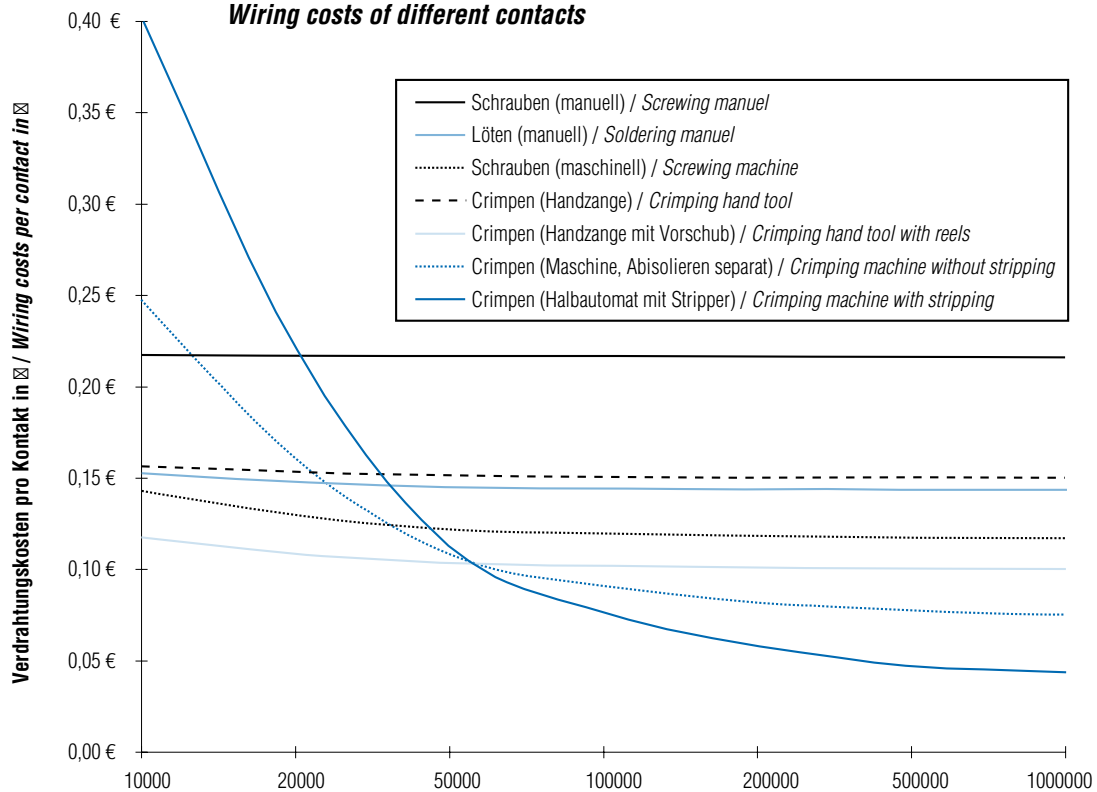
Verdrahtungskosten verschiedener Anschlussarten Wiring costs of different contacts
